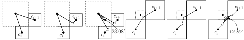
Fig. 13: s_i : s : s_{i+1} \equiv 1 : 2 : 1
