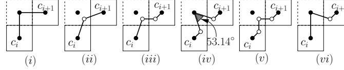
Fig. 12: s_i : s : s_{i+1} \equiv 1 : 1 : 1
